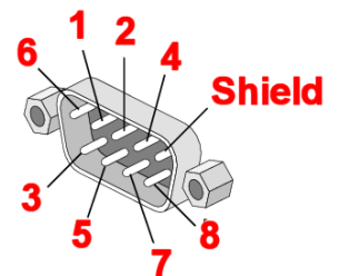
Pinbelegung des 9-Pin D-Sub Anschlusses
